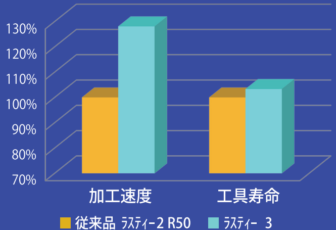
200mm #80 自社試験結果 バルチックキング 50x50cm 大和自動
